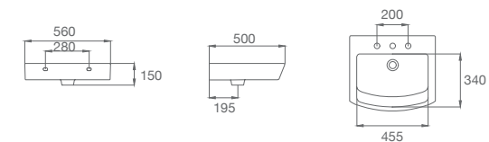
HALL 550 Medidas: 560 x 500 mm. Incluye juego de fijación. No incluye grifería. 1230030001200 1 orificio 1230030003200 3 orificios
