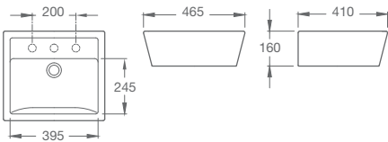
SENDAI Medidas: 465 x 410 x 160 mm. No incluye grifería. 1420320001200 1 orificio 1420320003200 3 orificios
