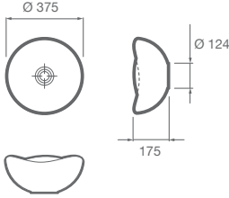
RUY OHTAKE 375 Medidas: Ø 375 x 175 mm. Fineceramic®. Incluye tapón fijo abierto de porcelana. No incluye desagüe. A327A15620 A327A15640 A327A15660 A327A15870
