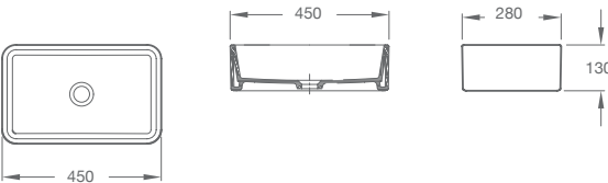
LEA RECTANGULAR Medidas: 450 x 280 x 130 mm. Sin orificios. Admite grifería de caño alto o de pared. 1400400000200
