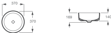
INSPIRA ROUND Medidas: Ø 370 x 140 mm. Fineceramic®. Incluye desagüe con tapón fijo abierto de porcelana. A327523000
