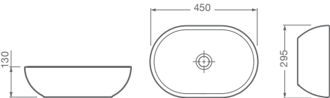
LEA OVAL Medida: 450 x 295 x 130 mm. Sin orificios. Admite grifería de caño alto o de pared. 1400410000200
