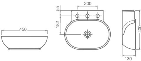
LEA PLUS Medida: 450 x 400 x 130 mm. Se suministra con 1 orificio central practicado y 2 insinuados. No incluye grifería. A327A1F000
