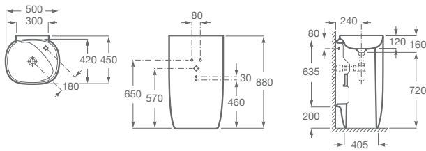
BEYOND Medidas: 500 x 880 mm. Fineceramic®. Se suministra con 1 orificio del lado derecho. Incluye desagüe universal con tapón cerámico Ø 72 mm. No incluye grifería. A3270B0000
