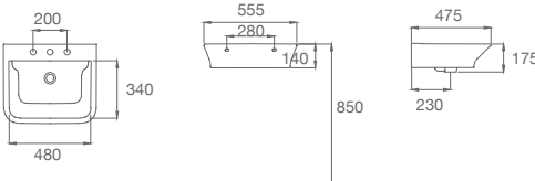
THE GAP 550 Medidas: 555 x 475 mm. Incluye juego de fijación. No incluye grifería. 1110030001200 1 orificio 1110030003200 3 orificios
