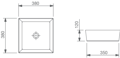
KIRA SQUARE Medidas: 380 x 380 x 120 mm. Sin orificios. Admite grifería de caño alto o de pared. A327A1G000 A327A1G000
