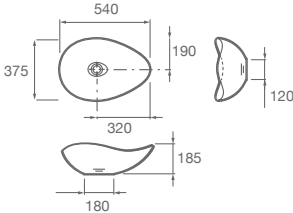
RUY OHTAKE 540 Medidas: 540 x 375 x 185 mm. Fineceramic®. Incluye tapón fijo abierto de porcelana. No incluye desagüe. A327A13620 A327A13640 A327A13660
