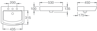
HALL 520 Medida: 530 x 450 mm. No incluye grifería. 1230370001200 1 orificio 1230370003200 3 orificios
