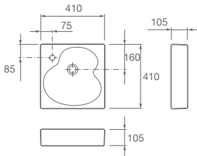
RUY OHTAKE 410 Medidas: 410 x 410 x 105 mm. No incluye tapón cerámico, desagüe ni grifería. A327A14620 A327A14640 A327A14860
