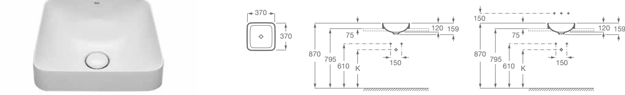
BACHA SQUARE / ENCIMERA A32753R000 Medidas: 370 x 370 x 120 mm. Incluye desagüe con tapón fijo abierto de porcelana. Finceramic®
