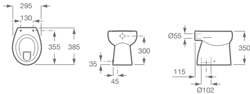
INODORO PARA NIÑOS BABY A344PB8000 Inodoro para niños. Salida vertical. Incluye juego de fijación. A801PB6004 Asiento Baby para inodoro infantil.
