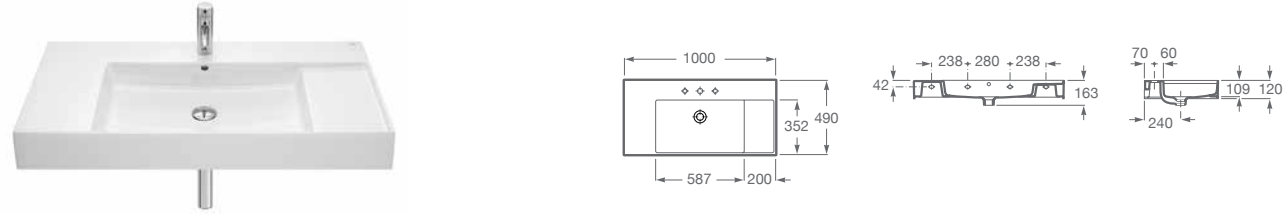
BACHA 1000 / SOBRE ENCIMERA / MURAL A32752A000 Medidas: 1000 x 490 x 120 mm. Se suministra con 1 orificio central practicado y 2 insinuados. Incluye juego de fijación. No incluye desagüe ni grifería. Finceramic®
