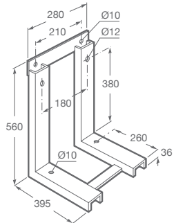
SOPORTE BASTIDOR c Soporte bastidor para inodoro y bidé suspendido. Incluye fijaciones. Set de montaje para pared (mínimo 15 cm.)
