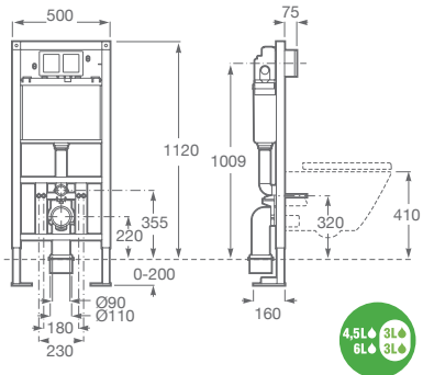
WC FREESTANDING A890090700 Estructura empotrable con depósito de doble descarga. Incluye accesorios de instalación con fijaciones. Ver placas de accionamiento en página 48.
