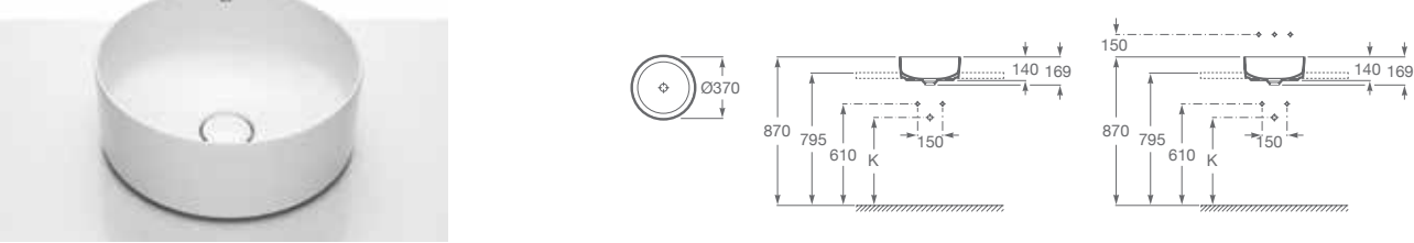
BACHA ROUND / SOBRE ENCIMERA A327523000 Medidas: Ø 370 x 140 mm. Incluye desagüe con tapón fijo abierto de porcelana. Finceramic®
