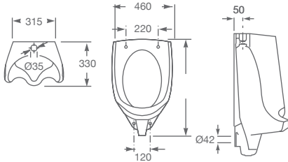
URINARIO 3521720000200 Urinario con entrada de agua superior. No incluye grifería. Se expide con tapón de limpieza, juego de fijación, manguito y enchufe de alimentación. Opcional: codo de fundición, empotrable para desagüe.
