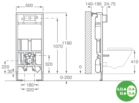
WC SMART A890090800 Soporte para inodoro In-Wash suspendido. Estructura empotrable con depósito de doble descarga. Incluye accesorios de instalación con fijaciones. Ver placas de accionamiento en página 48.
