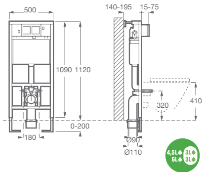
WC DUPLO A890090020 Bastidor con depósito empotrable de doble descarga para inodoro suspendido. Codo de 90° / 110° Ver placas de accionamiento página 48.
