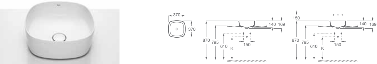
BACHA SOFT / SOBRE ENCIMERA A327502000 Medidas: 370 x 370 x 140 mm. Incluye desagüe con tapón fijo abierto de porcelana. Finceramic®
