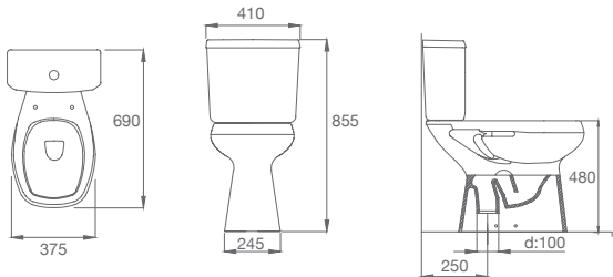
INODORO LARGO Y DEPÓSITO 1066100000202 Salida vertical. Incluye juego de fijación, asiento y tapa.
