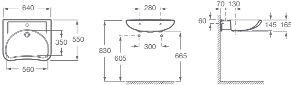
BACHA MURAL A327230000 Se suministra con 1 orificio practicado y 2 insinuados. Incluye juego de fijación. No incluye grifería.
